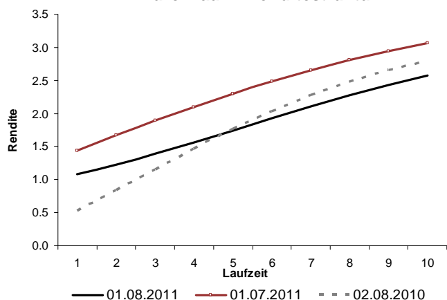
Euro-Raum: Renditestruktur
