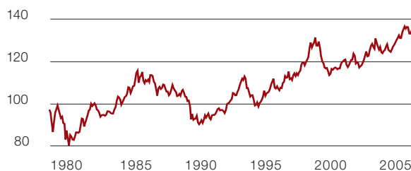
Kurse 10-jähriger deutscher Staatsanleihen in %
